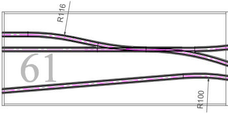
Modul nr. B-SMJK-61 Hovedspor og 3 sidespor Lengde: 120 cm Tema: Rognan Stasjon Del 5 av 7
