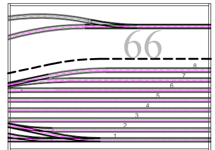
Modul nr. B-SMJK-66 Lengde hovedspor: 110 cm Tema: Feladalen
