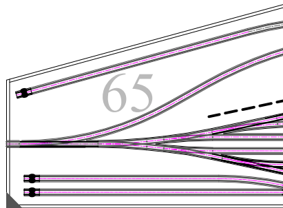
Modul nr. B-SMJK-65 Skinnelengde hovedspor: 111/117 cm Tema: Innkjøring Feladalen
