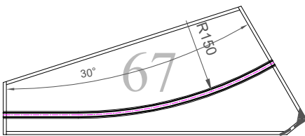
Modul nr. B-SMJK-67 Skinnelengde: 107 cm Tema: Feladalen rundbane
