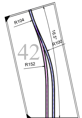
Modul nr. B-OF-42 Lengde hovedspor: 109 cm 1 sidespor og 1 hovedspor Tema: Sidespor med sagbruk
