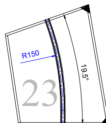
Modul nr. B-JHT-23 Skinnelengde hovedspor: 60 cm Hovedspor krysser en bekk Tema: Tidligere ved Oteråga Stasjon
