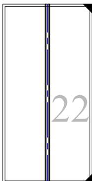
Modul nr. B-HJP-22 Skinnelengde hovedspor: 100 cm Avkjørsel til Reitan - bru over hovedspor Tema: Oteråga Stasjon
