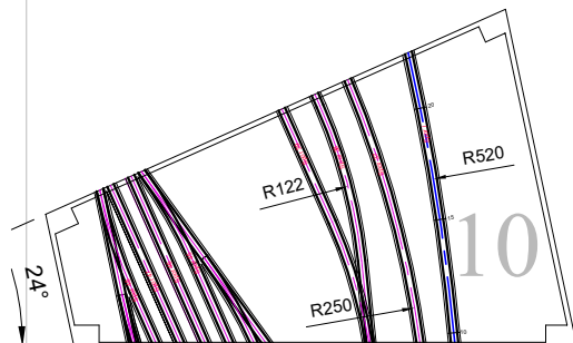
Modul nr. B-SMjK-10 Skinnelengde hovedspor: 71 cm Stigning: 1,86 % 10 sidespor + 1 hovedspor Tema: Bodø Stasjon
