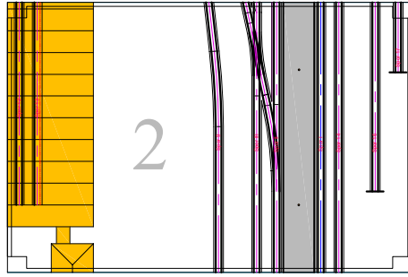
Modul nr. B-SMjK-2 Skinnelengde hovedspor: 80 cm 4 sidespor, perong og 3 hovedspor Tema: Bodø Stasjon
