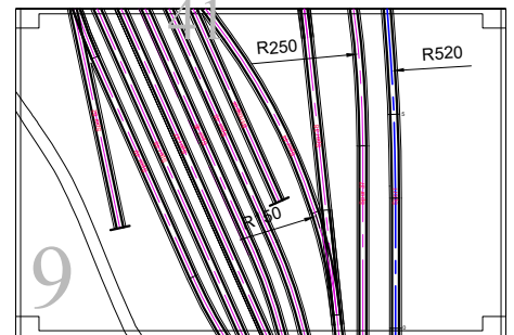
Modul nr. B-SMjK-9 Skinnelengde hovedspor: 80 cm, start stigning 10 sidespor + 1 hovedspor Tema: Bodø Stasjon
