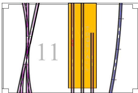
Modul nr. B-SMjK-11 Skinnelengde hovedspor: 81 cm Stigning 1,86 % 7 sidespor + 1 hovedspor Tema: Lokstall Bodø Stasjon
