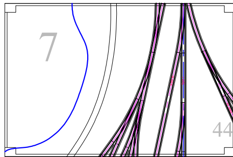
Modul nr. B-SMjK-7 Skinnelengde hovedspor: 80 cm 7 sidespor og 3 hovedspor Tema: Bodø Stasjon
