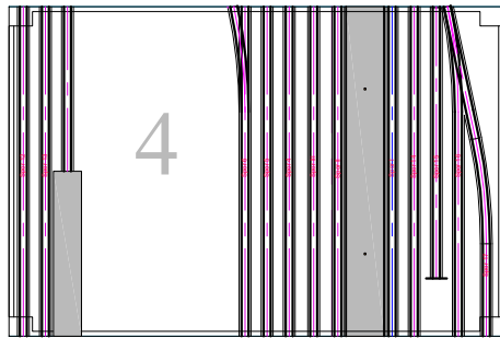
Modul nr. B-SMjK-4 Skinnelengde hovedspor: 80 cm 9 sidespor, perong og 3 hovedspor Tema: Bodø Stasjon
