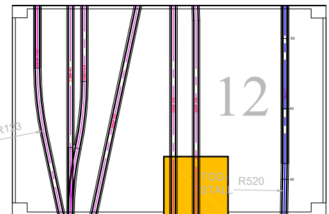
Modul nr. B-SMjK-12 Skinnelengde hovedspor: 80 cm Stigning 1,86 % 6 sidespor + 1 hovedspor Tema: Lokstall Bodø Stasjon
