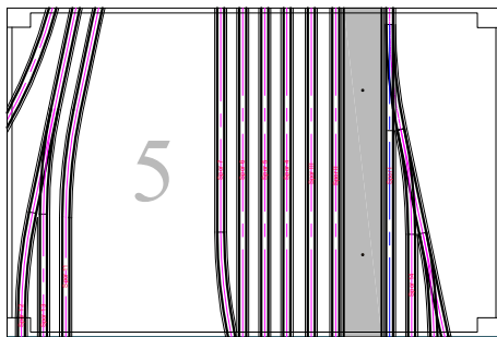
Modul nr. B-SMjK-5 Skinnelengde hovedspor: 80 cm 10 sidespor, perong og 3 hovedspor Tema: Bodø Stasjon
